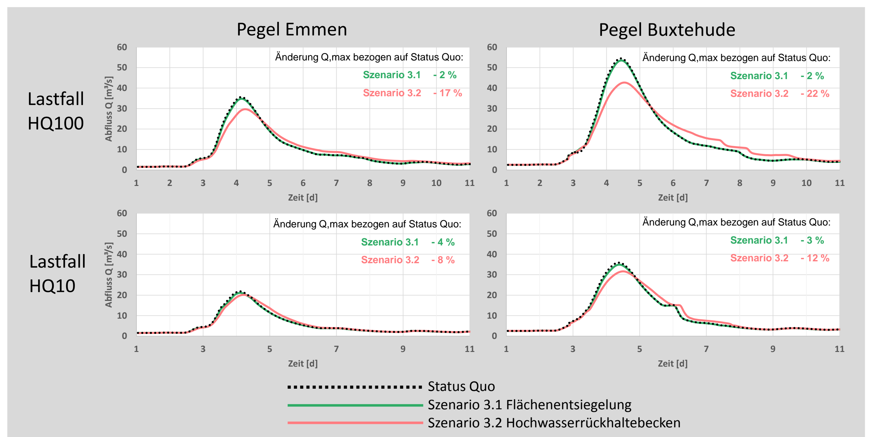
Abbildung 5: Änderung der Hochwasserabflusskurven für die Este aufgrund verschiedener Klimaanpassungsmaßnahmen; obere Zeile: Lastfall HQ100 (100-jährliches Ereignis); untere Zeile: Lastfall HQ10 (10-jährliches Ereignis); linke Spalte: Ganglinie am Pegel Emmen; rechte Spalte: Ganglinie am Pegel Buxtehude.
